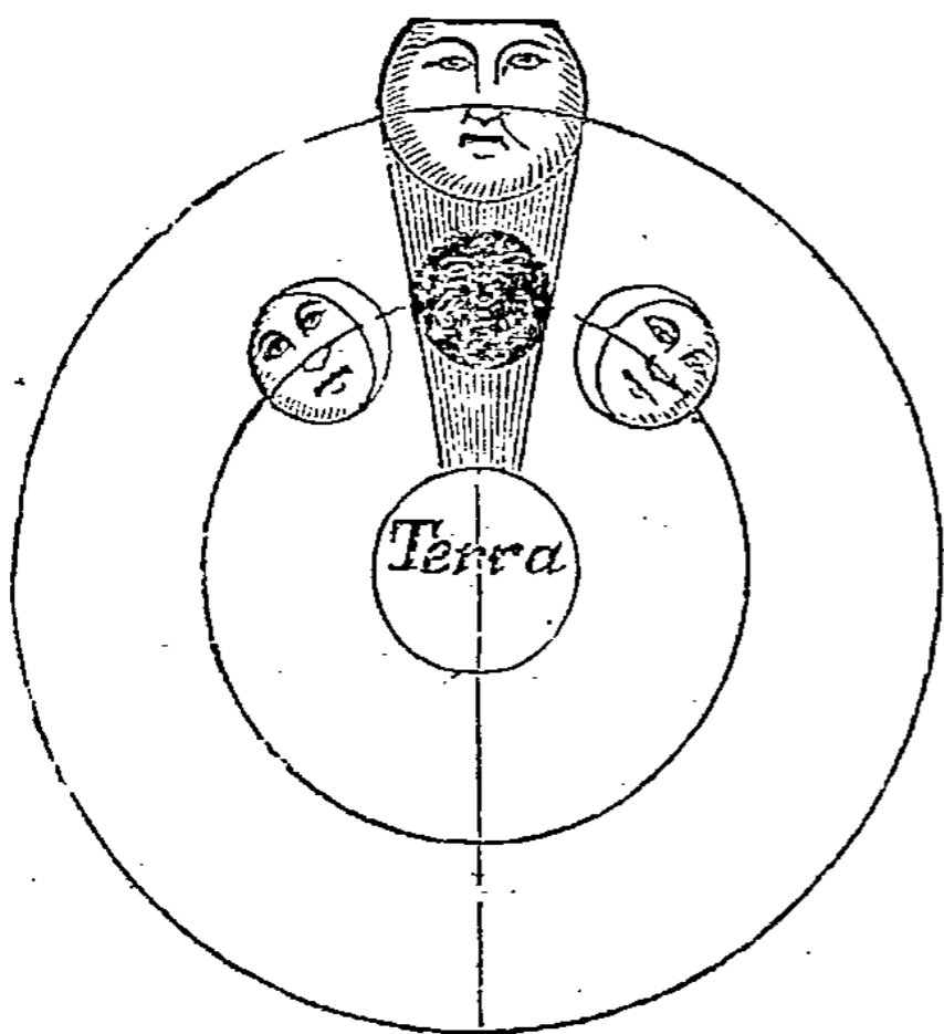
Eclipsis Solis.
